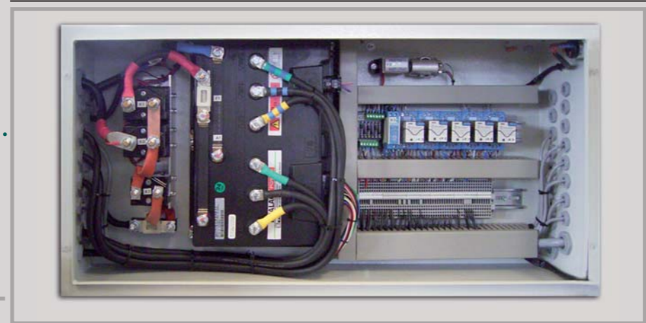
ATECH Schaltschrank mit Lenkrechner und allen Leistungsteilen, Schützen, Sicherungen und Klemmleisten
