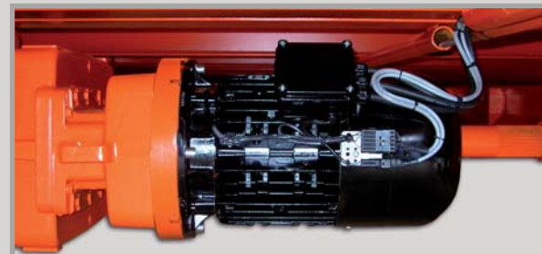
ATECH Drehstrom-Getriebeeinheiten für Doppelmotorantrieb
